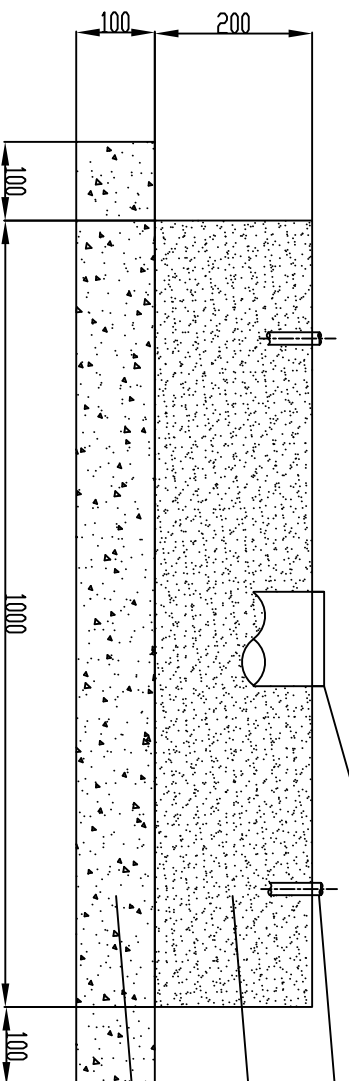
基础剖面图
